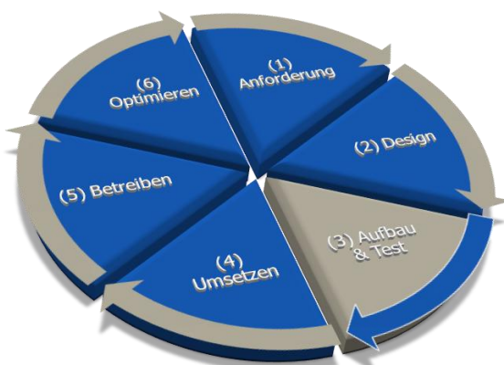
Software Lebenszyklus
